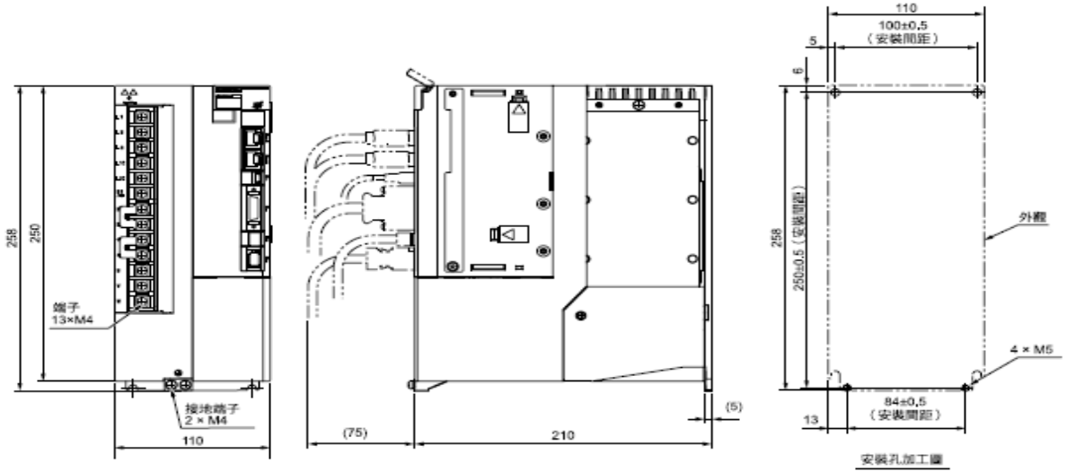
概略重量：4.4 kg 單位：mm
