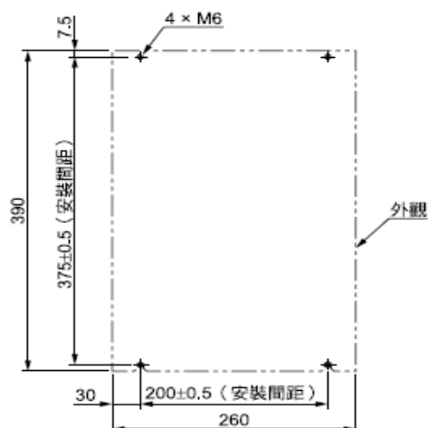
安裝孔加工圖
